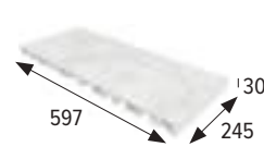
Rejilla cerámica oculta Hidden ceramic grid
