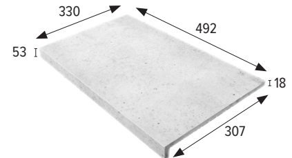
Peldaño recto 50 · Straight stair-tread 50
