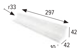
Rinconera transición Int. radial transition tile
