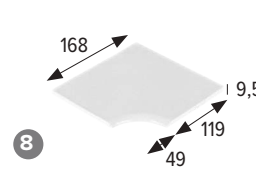
Esq. int. canto romo Bullnose int. corner
