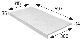
Peldaño recto 60 · Straight stair-tread 60
