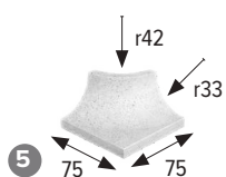
Esq. ext. cantonera External mitre
