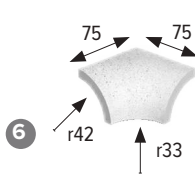
Esq. int. rinconera Internal mitre
