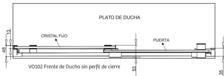
Dibujo Técnico
