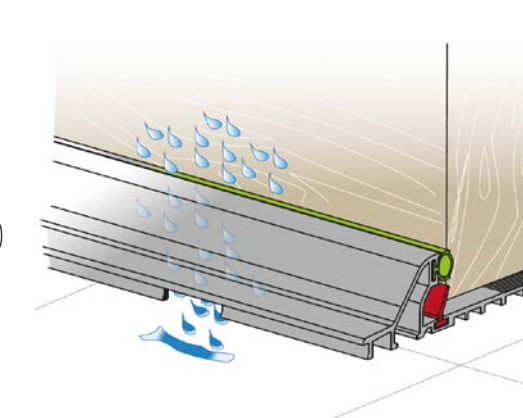
■ Perfil vierteaguas de aluminio (Sólo puertas abatibles)
